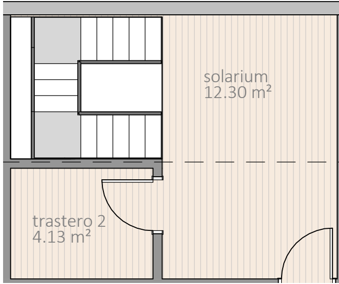
SOLARIUM-PLANTA CUBIERTA SUP. CONSTRUIDA: 16.5 m 2
